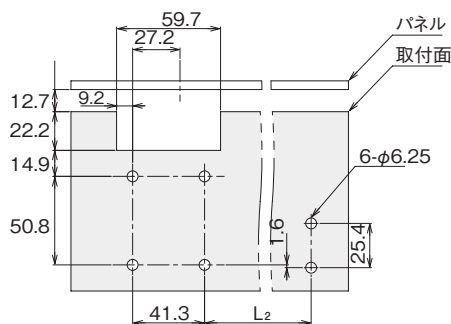
取付寸法
